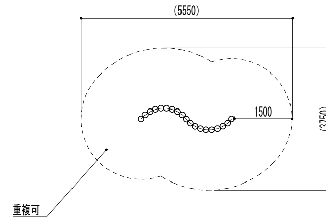
安全領域図 S=1/100
