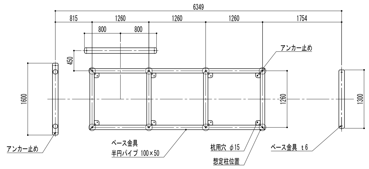
ベース金具伏図
