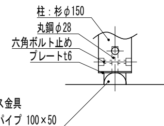
柱・ベース金具接続詳細図
