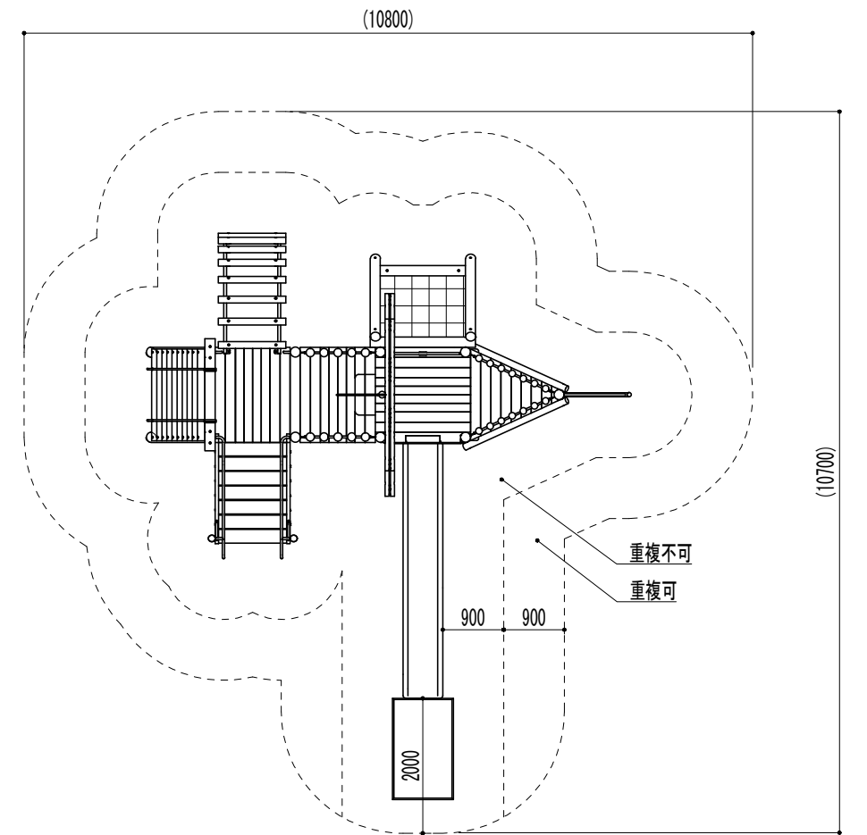
安全領域図 S=1/100
