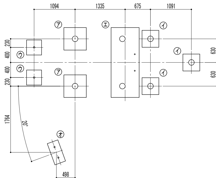
基礎伏図
