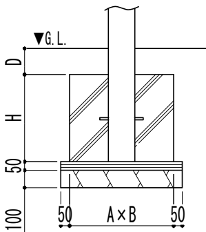
基礎詳細図
