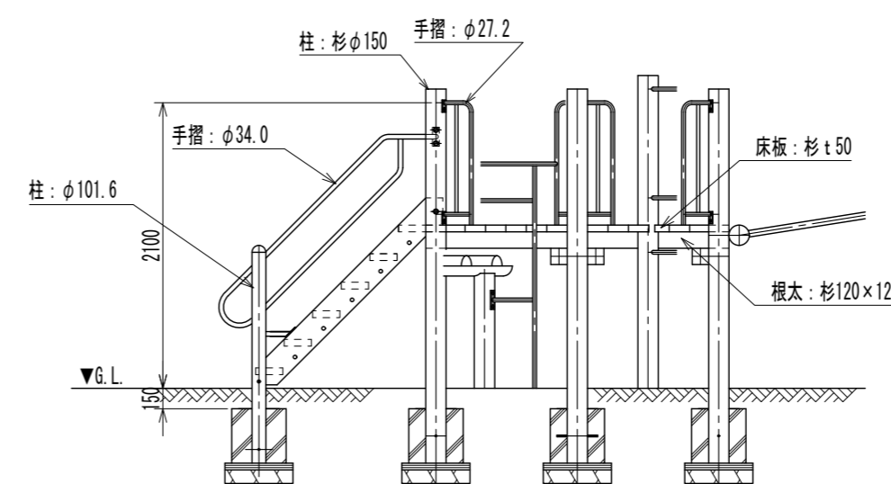
A-A 矢視図
