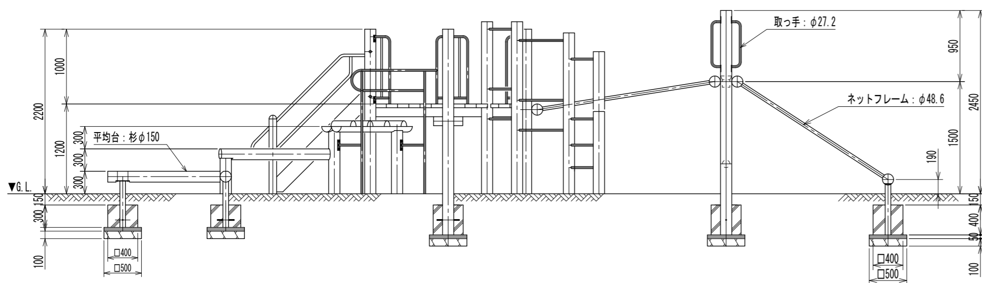
正面図
