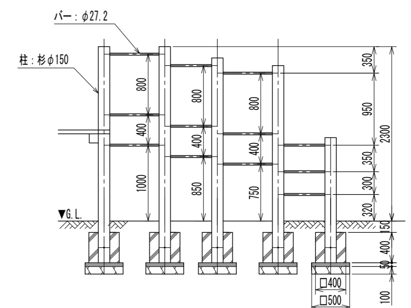
B-B 矢視図
