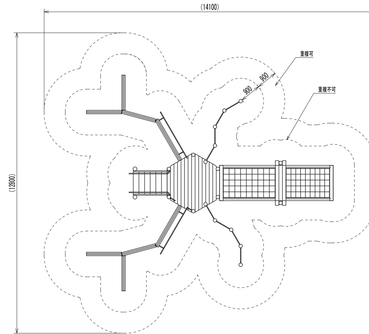
安全領域図 S=1/100
