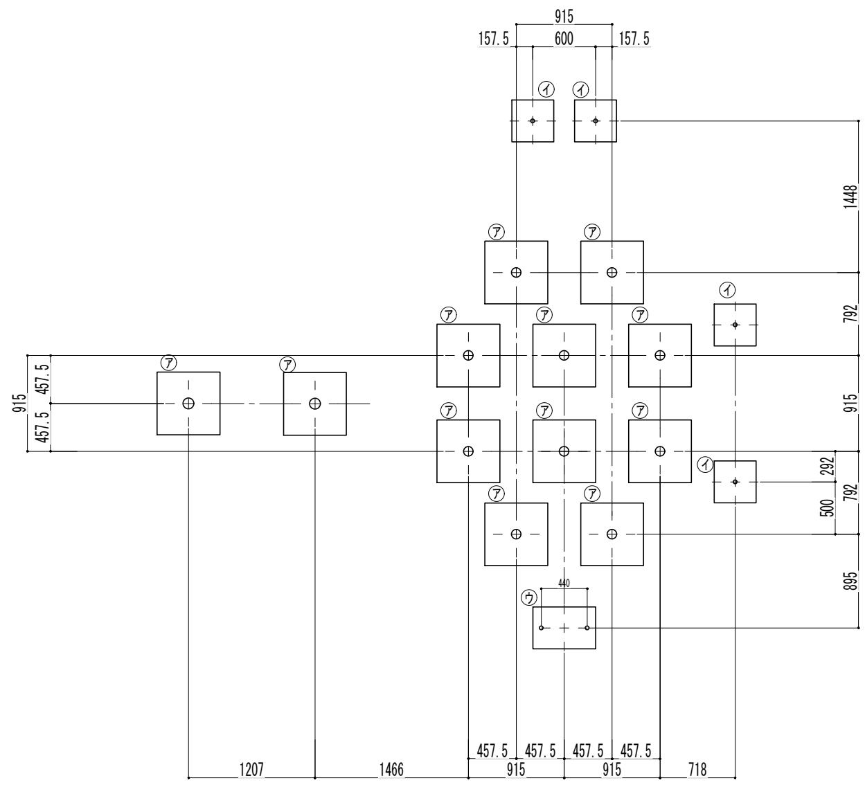
基礎伏図
