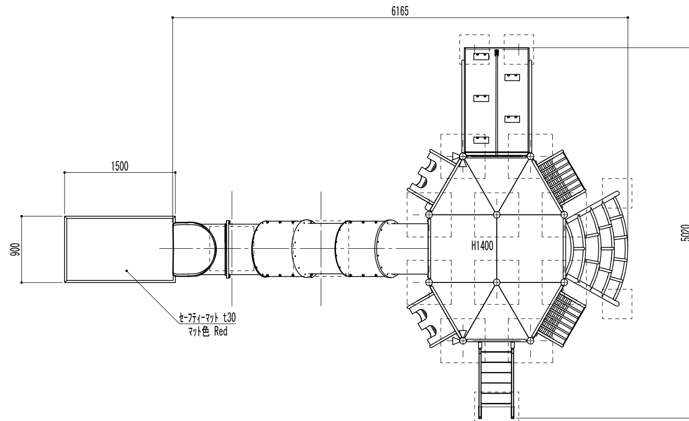
平面図
