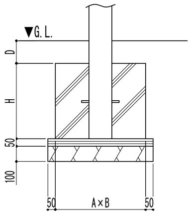
基礎詳細図
