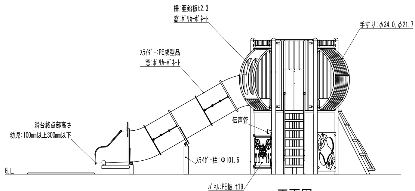
正面図
