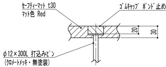
セーフティマット詳細図
