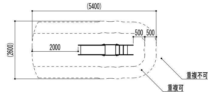
安全領域図 S=1/100
