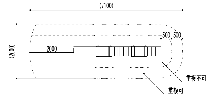
安全領域図 S=1/100
