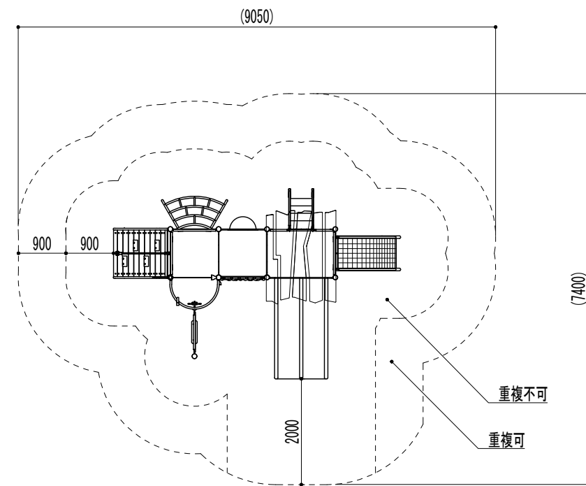
安全領域図 S=1/100
