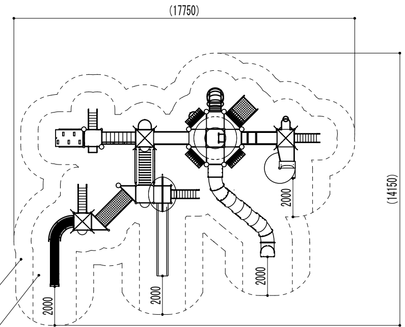
安全領域図 S=1/200
