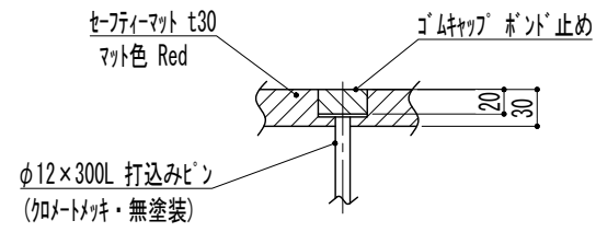
セーフティマット詳細図
