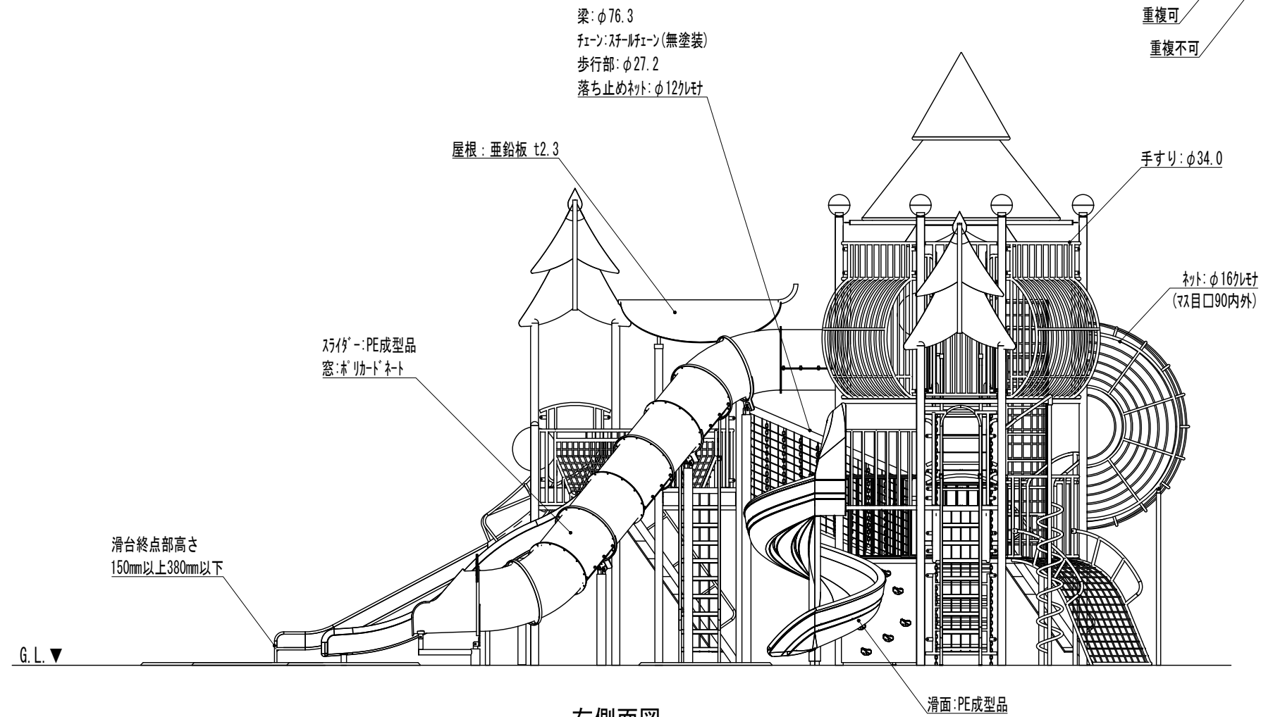
右側面図
