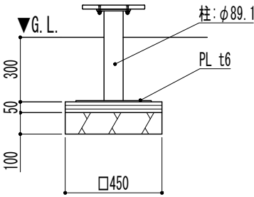
固定ステップ部 詳細図
