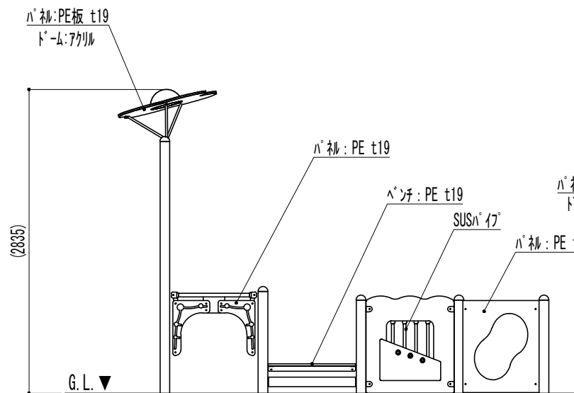
A-A (1:50)
