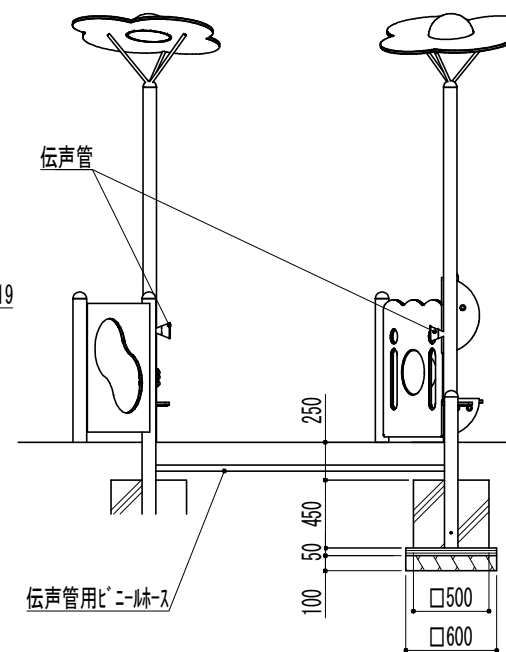
C-C (1:50)
