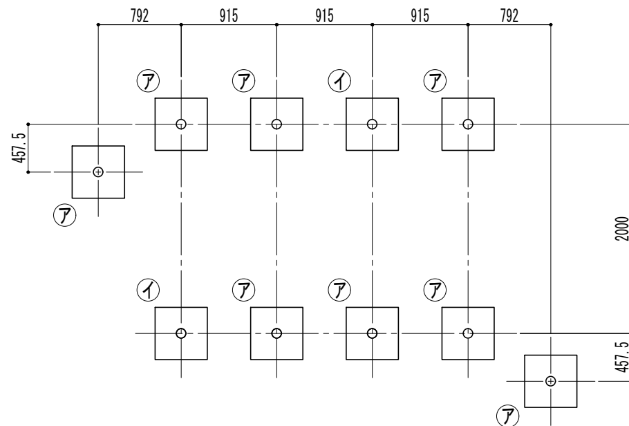
基礎伏図
