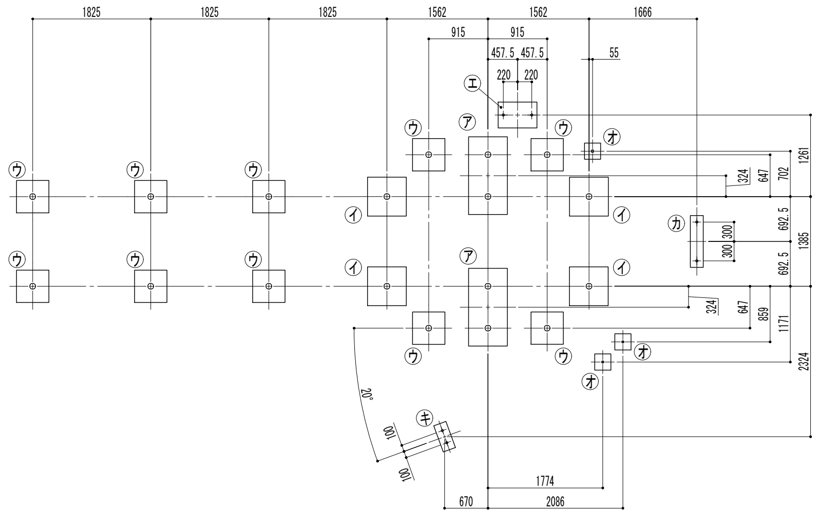
基礎伏図
