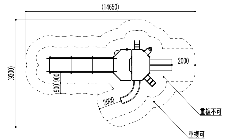
安全領域図 S=1/200
