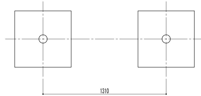
基礎伏図
