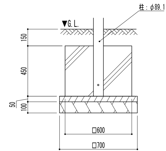
基礎詳細図
