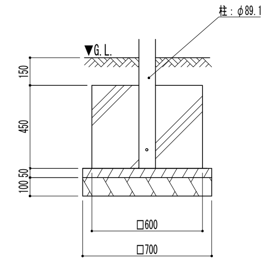
基礎詳細図
