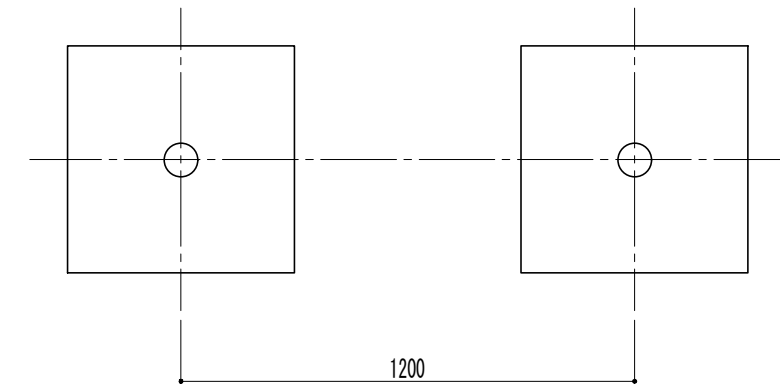
基礎伏図
