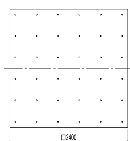
基礎伏図 S=1/30
