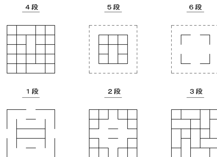
平面図 S=1/100
