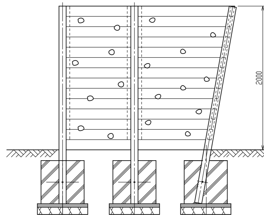
側面図 S=1/30
