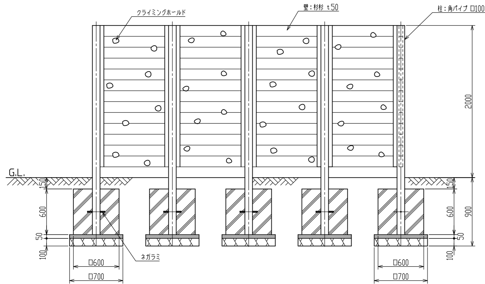
正面図 S=1/30
