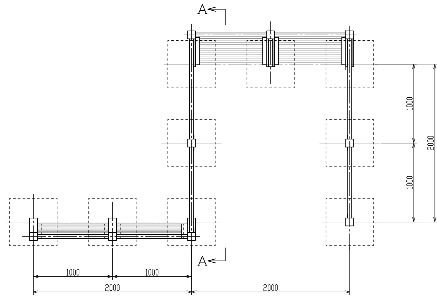
平面図 S=1/30
