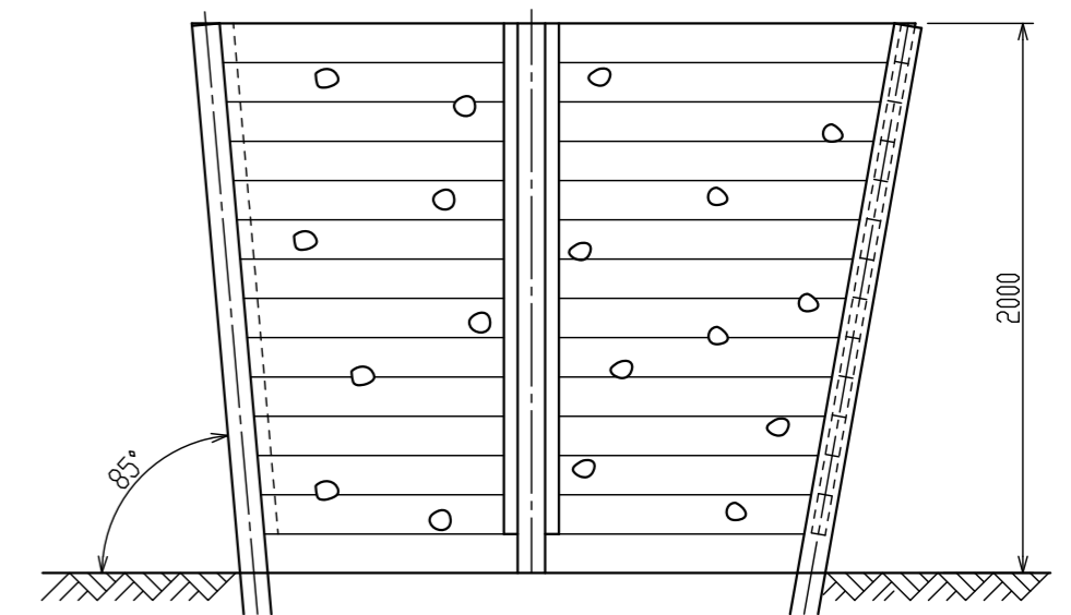
A-A矢視図 S=1/30
