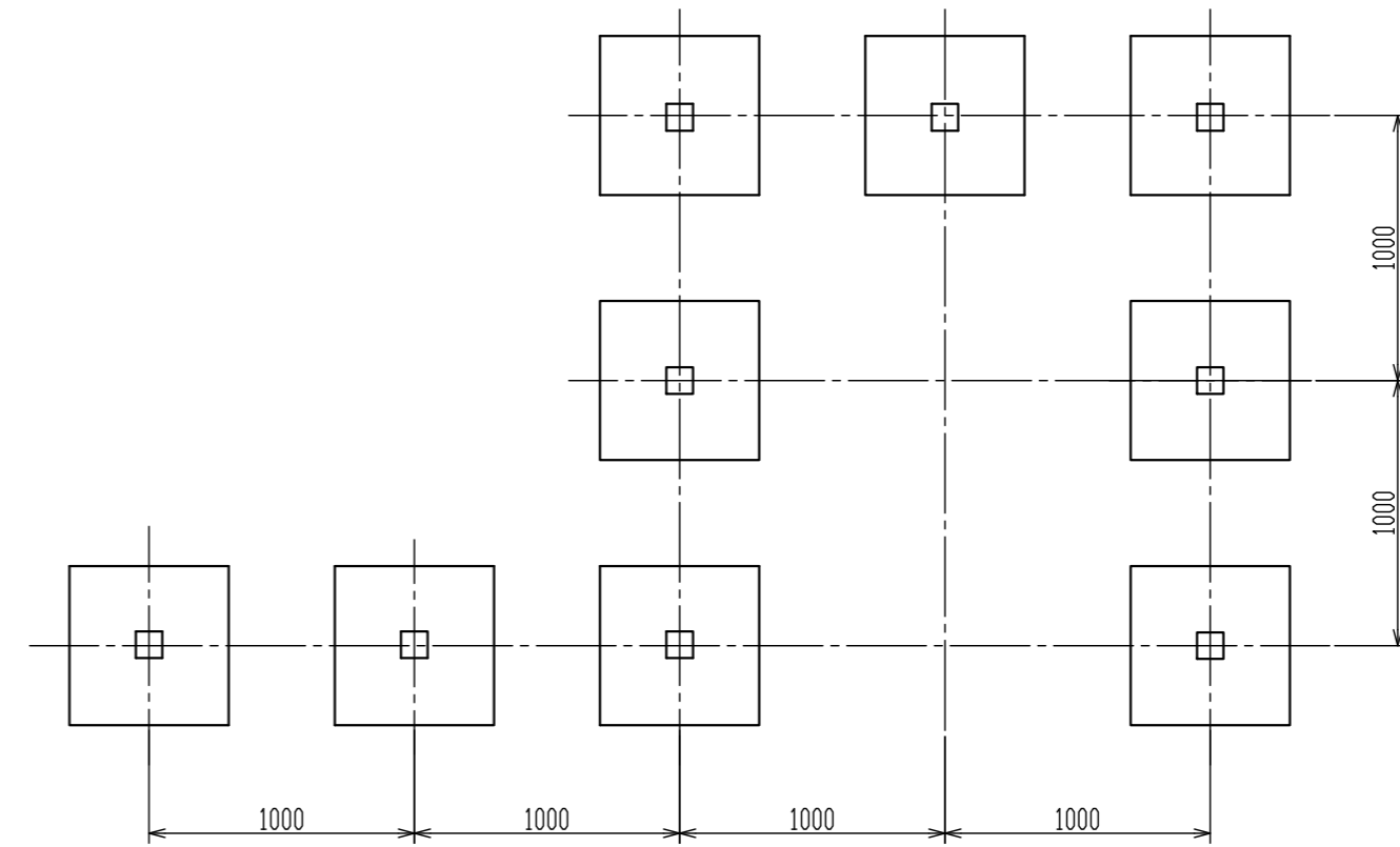
基礎伏図
