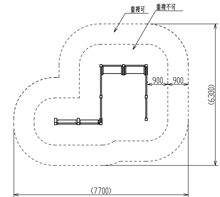
安全領域図 S=1/100
