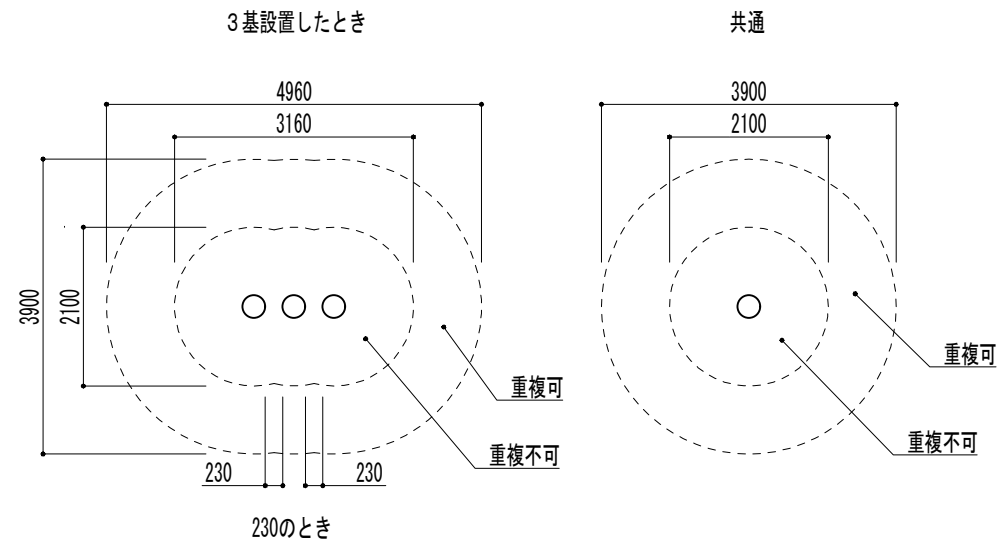
安全領域図
