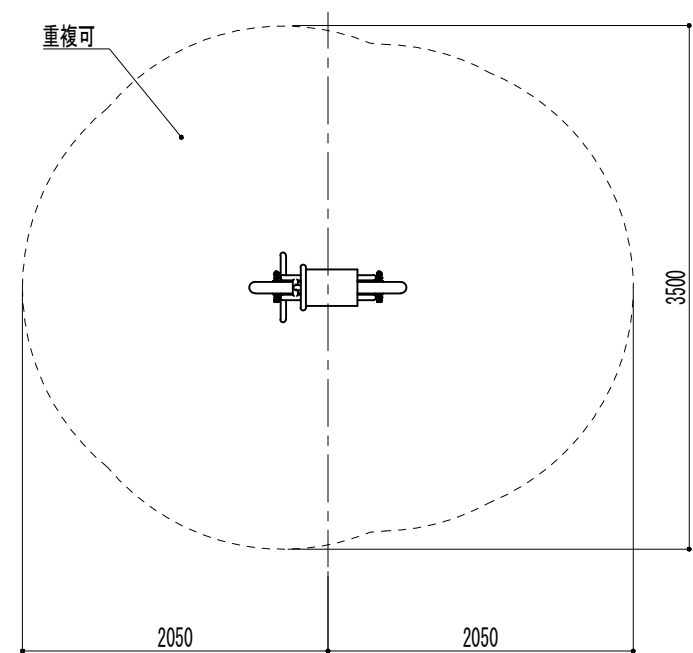
安全領域図S=1/50
