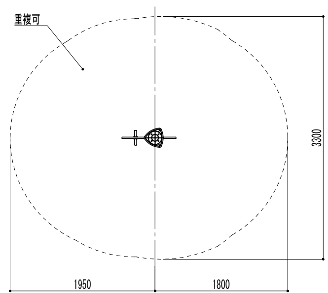
安全領域図S=1/50
