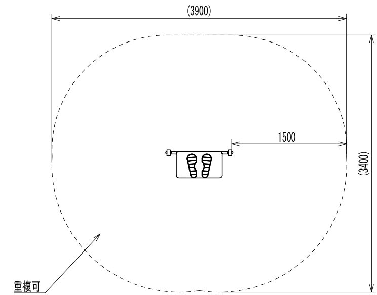
安全領域図 S=1/50
