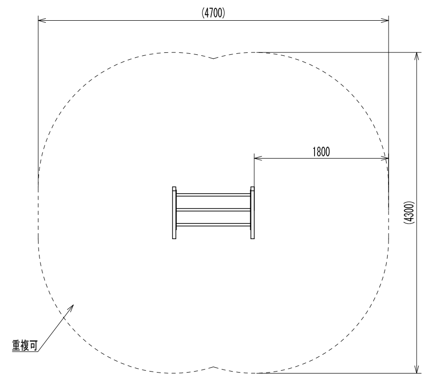
安全領域図 S=1/50
