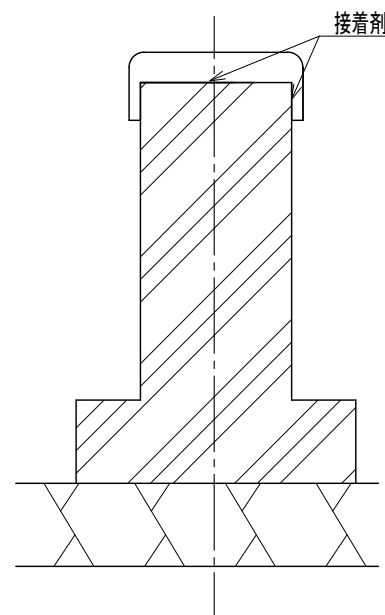
施工参考図
