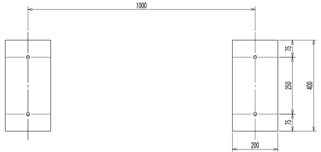
基礎伏せ図
