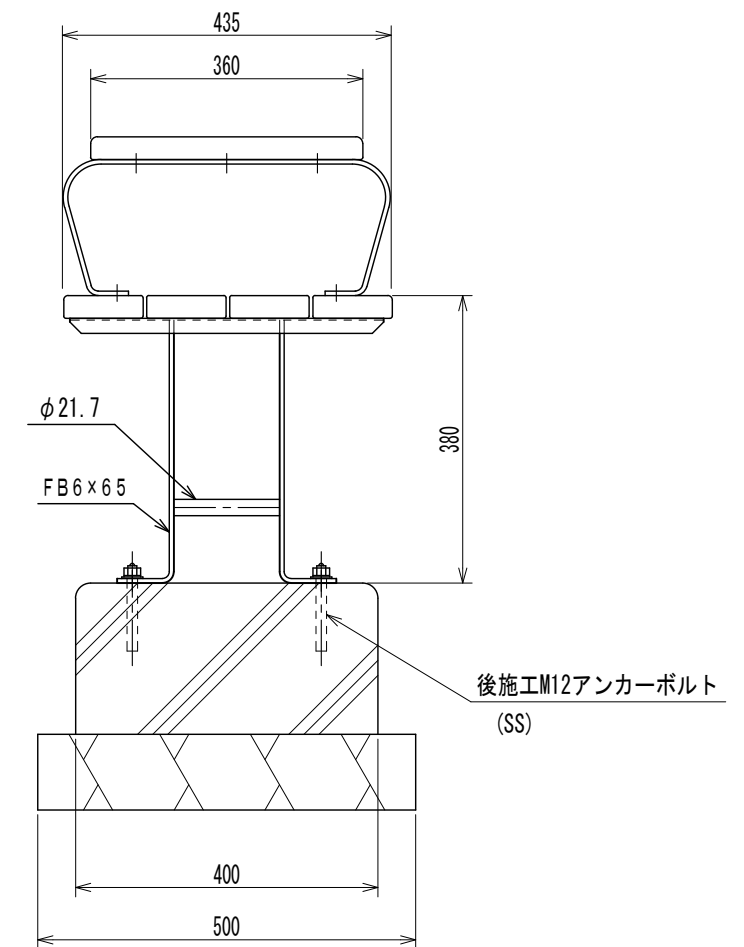
基礎伏せ図
