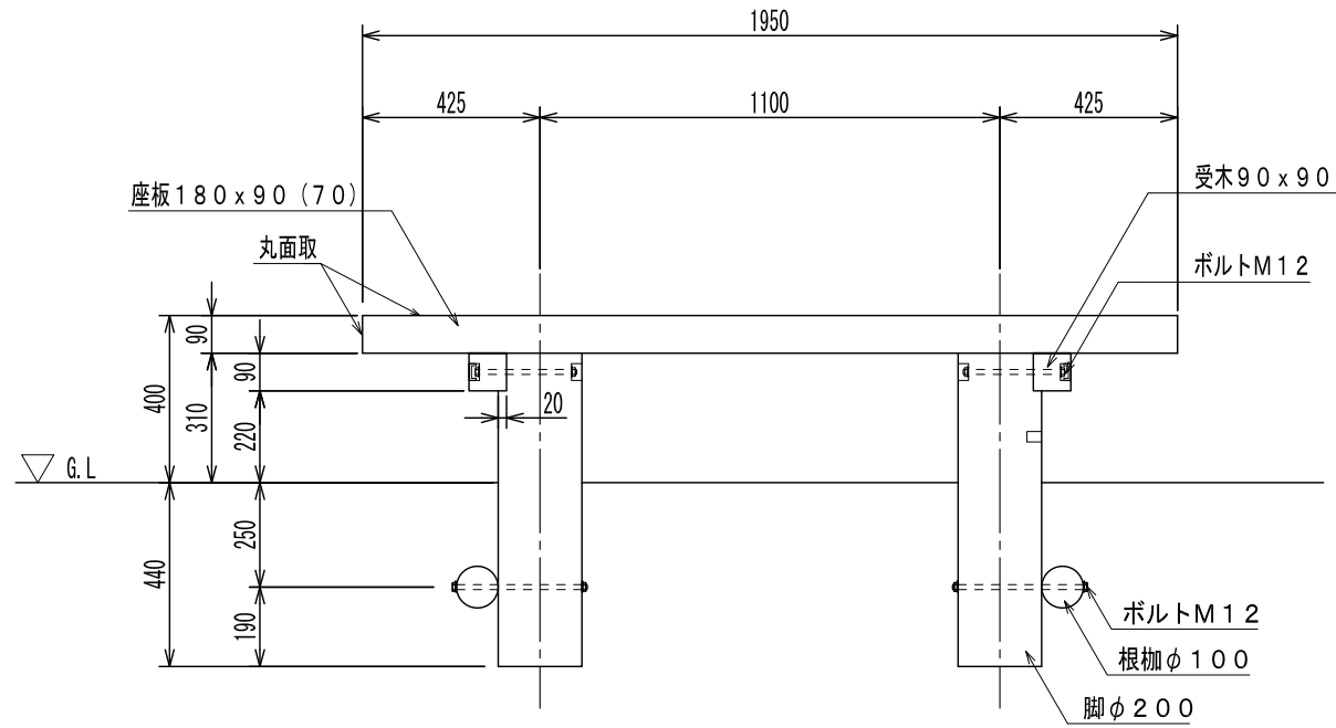
正面図
