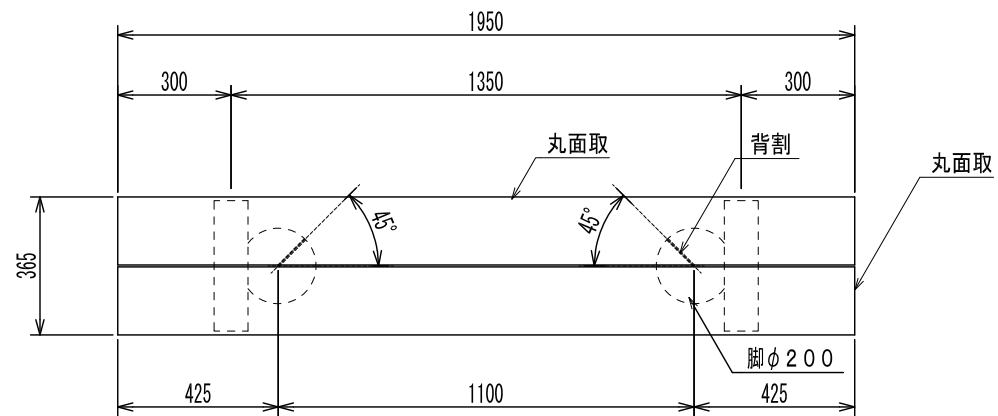
平面図
