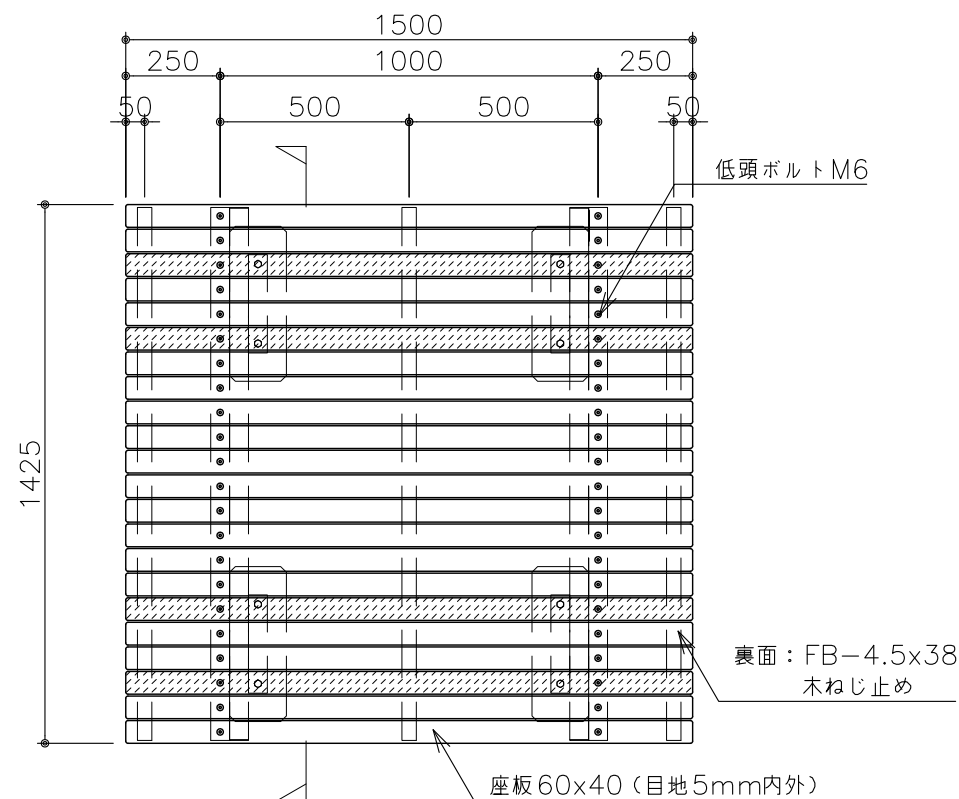
平面図 S=1:20
