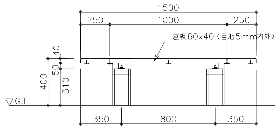
立面図 S=1:20
