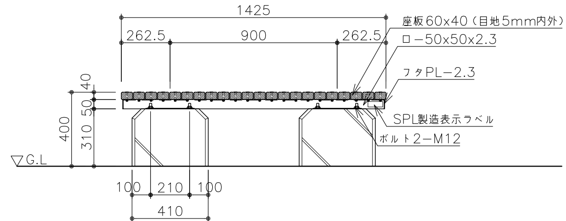
断面図 S=1:20
