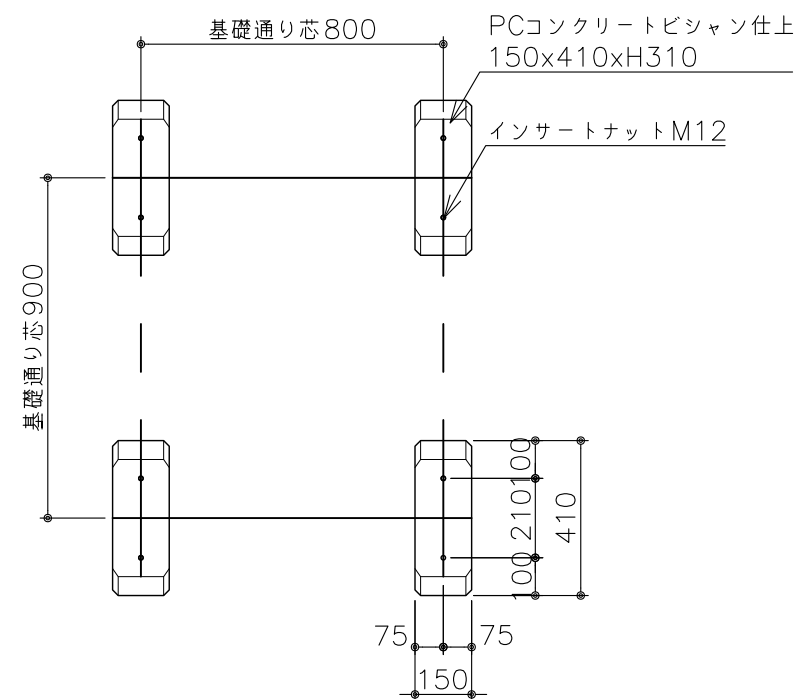
基礎伏図 S=1:20
