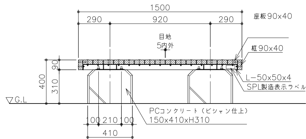
断面図 S=1:20
