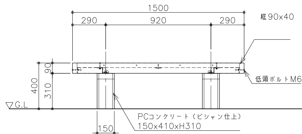
正面図 S=1:20
