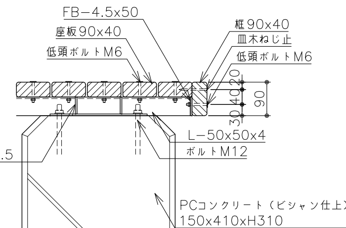
詳細図 S=1:10
