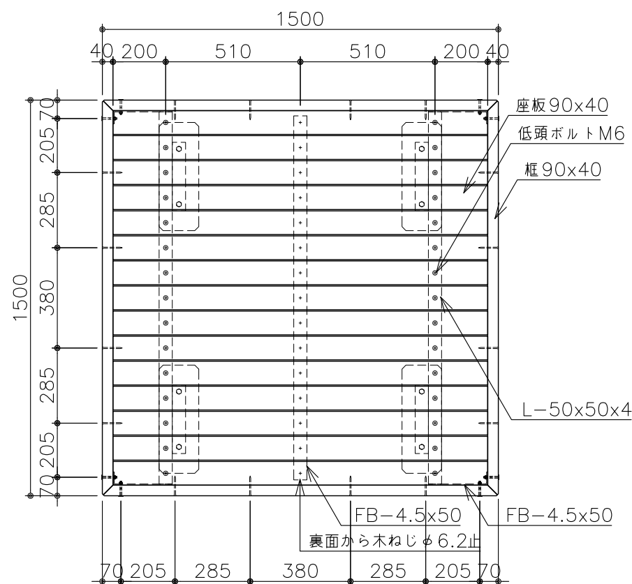
正面図 S=1:20
