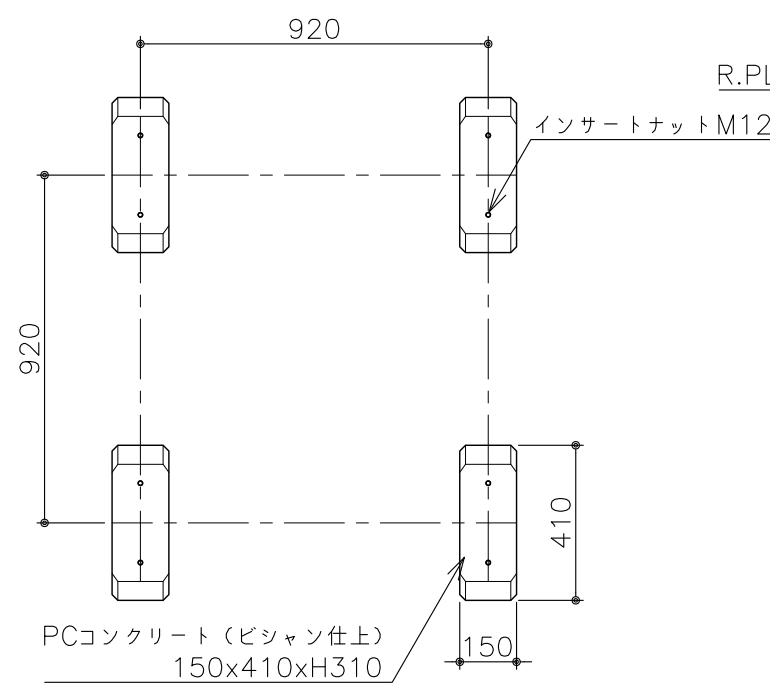
基礎伏図 S=1:20
