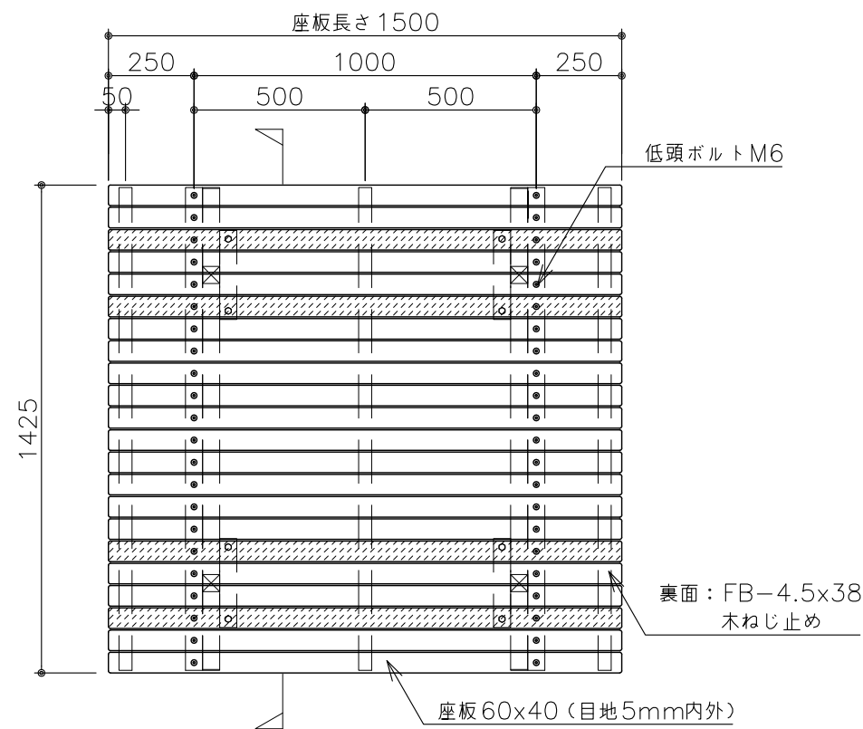
平面図 S=1:20
