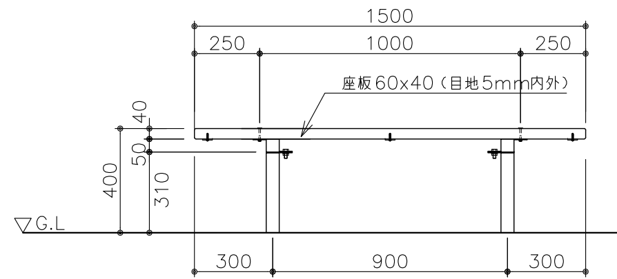
立面図 S=1:20
