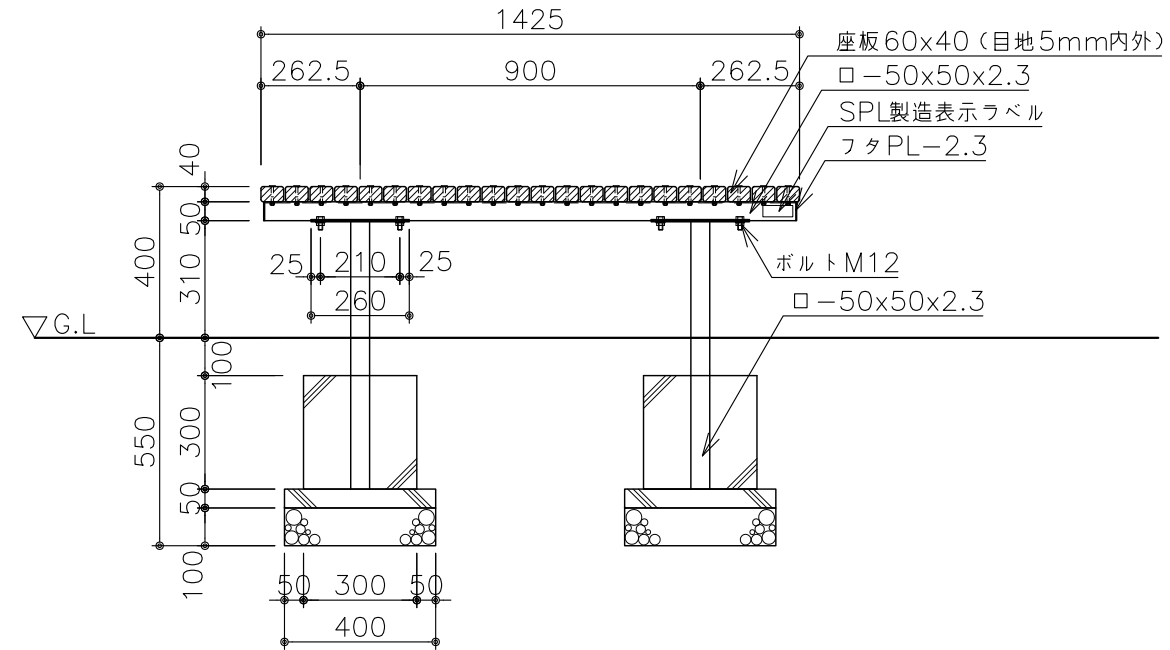
断面図 S=1:20
