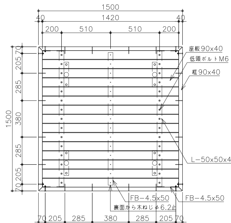
平面図 S=1:20
