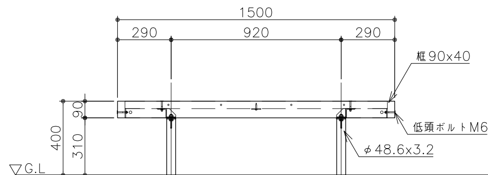
正面図 S=1:20
