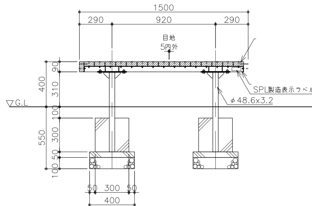
断面図 S=1:20
