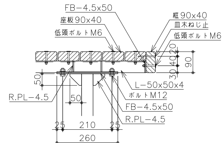
詳細図 S=1:10
