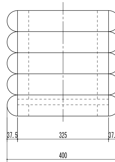
B矢視図 S=1/8
