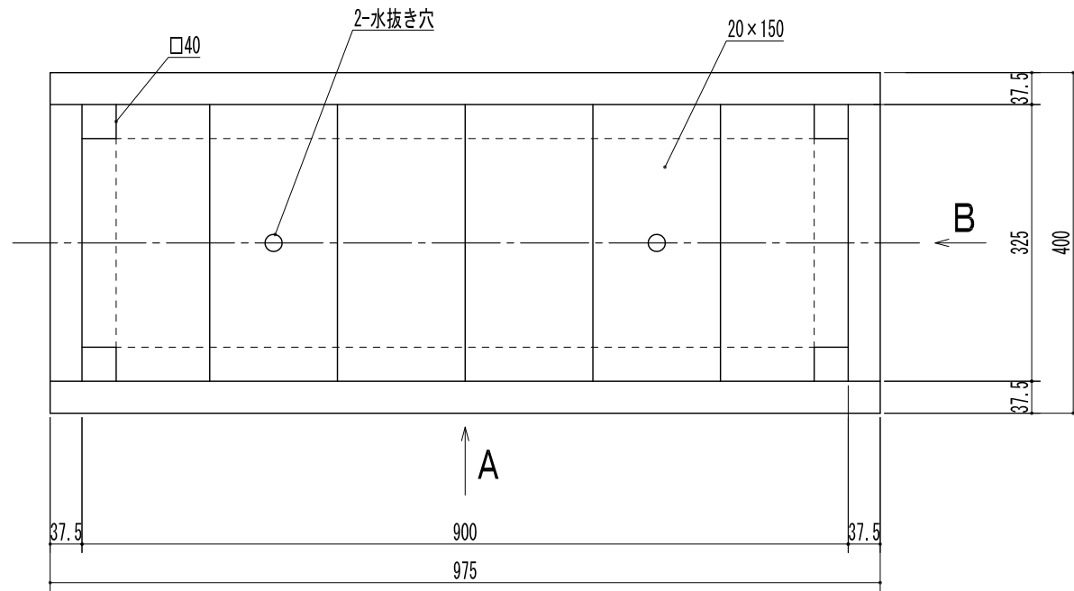
平面図 S=1/8
