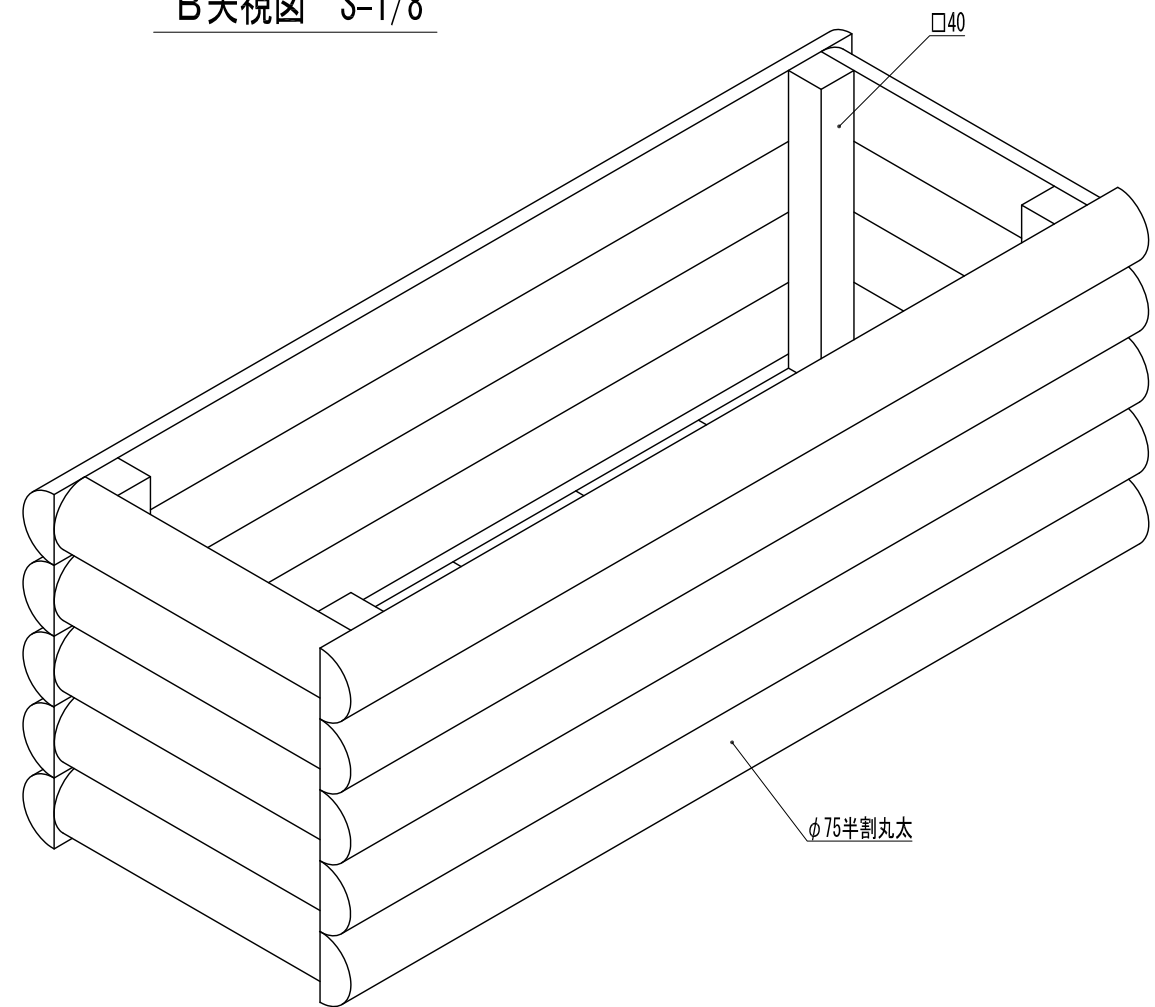
B矢視図 S=1/8
