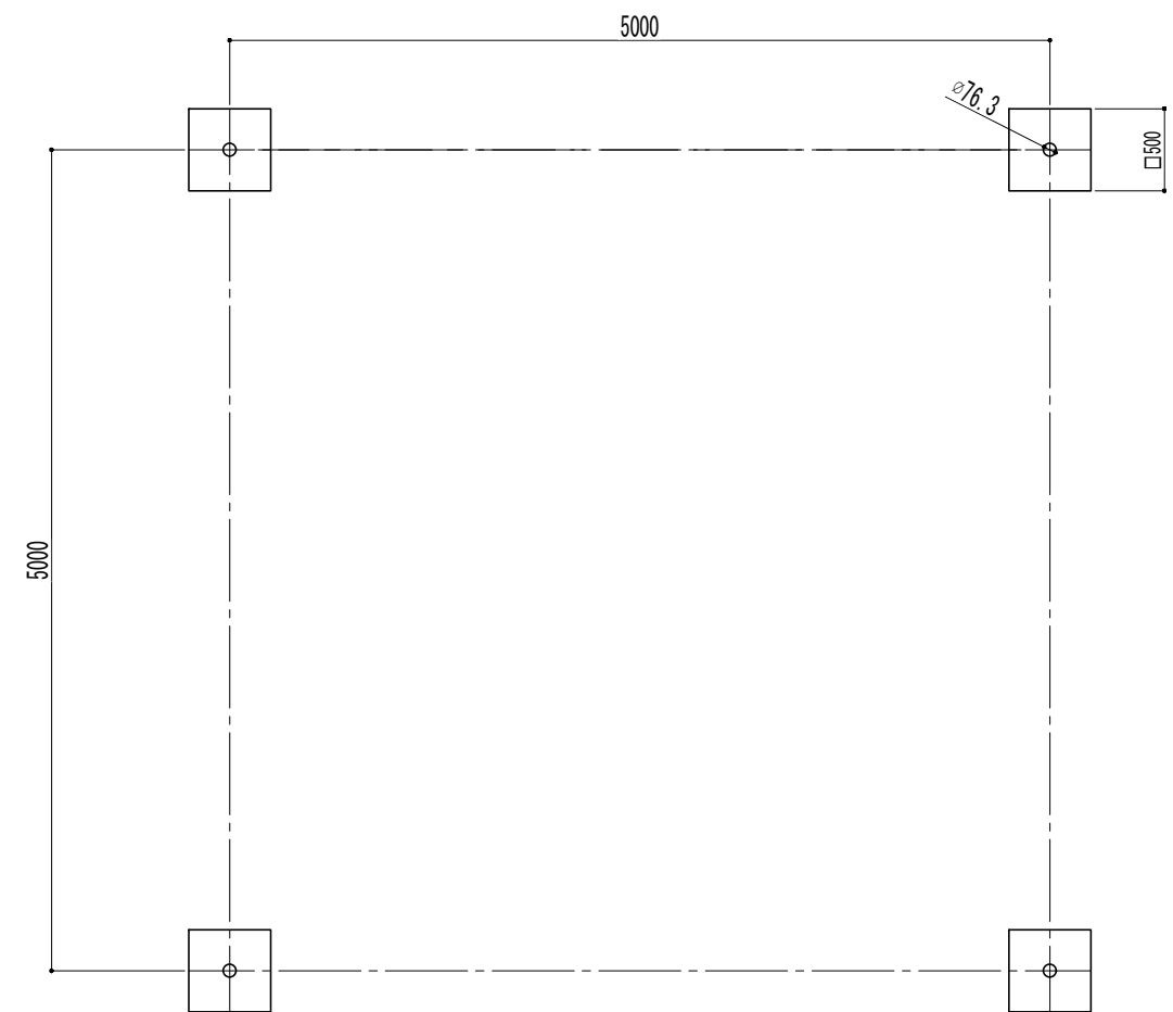
基礎伏図
