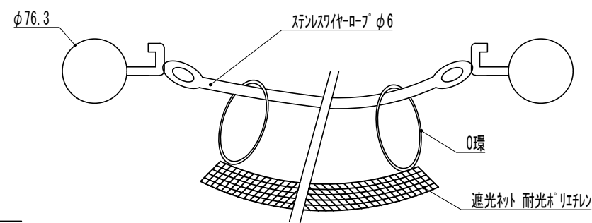
ワイヤーロープ 取付け部詳細 S=1:5
