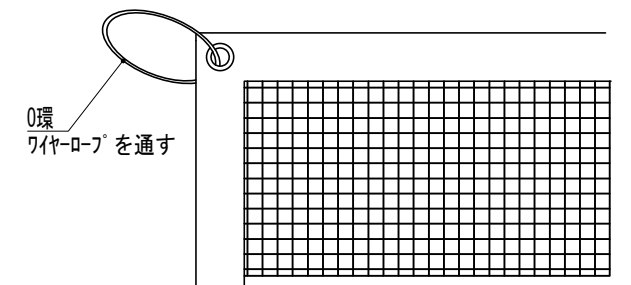
遮光ネット取付け部詳細 S=1:5
