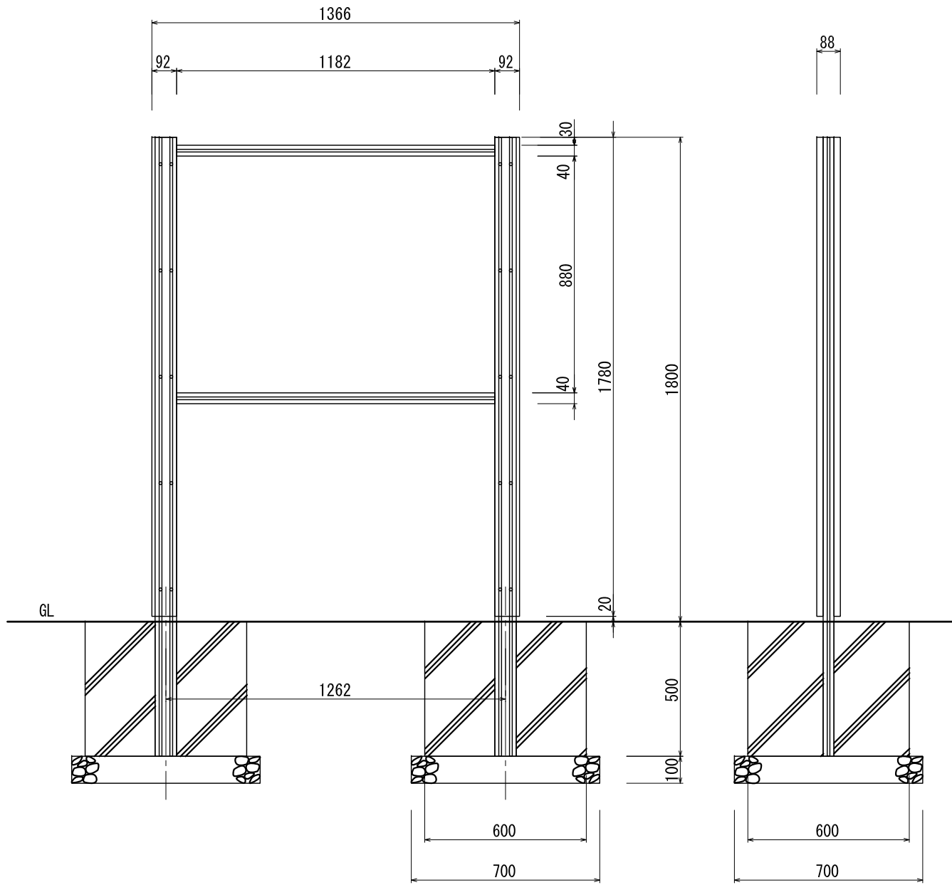
【正面図 S=1:20】
