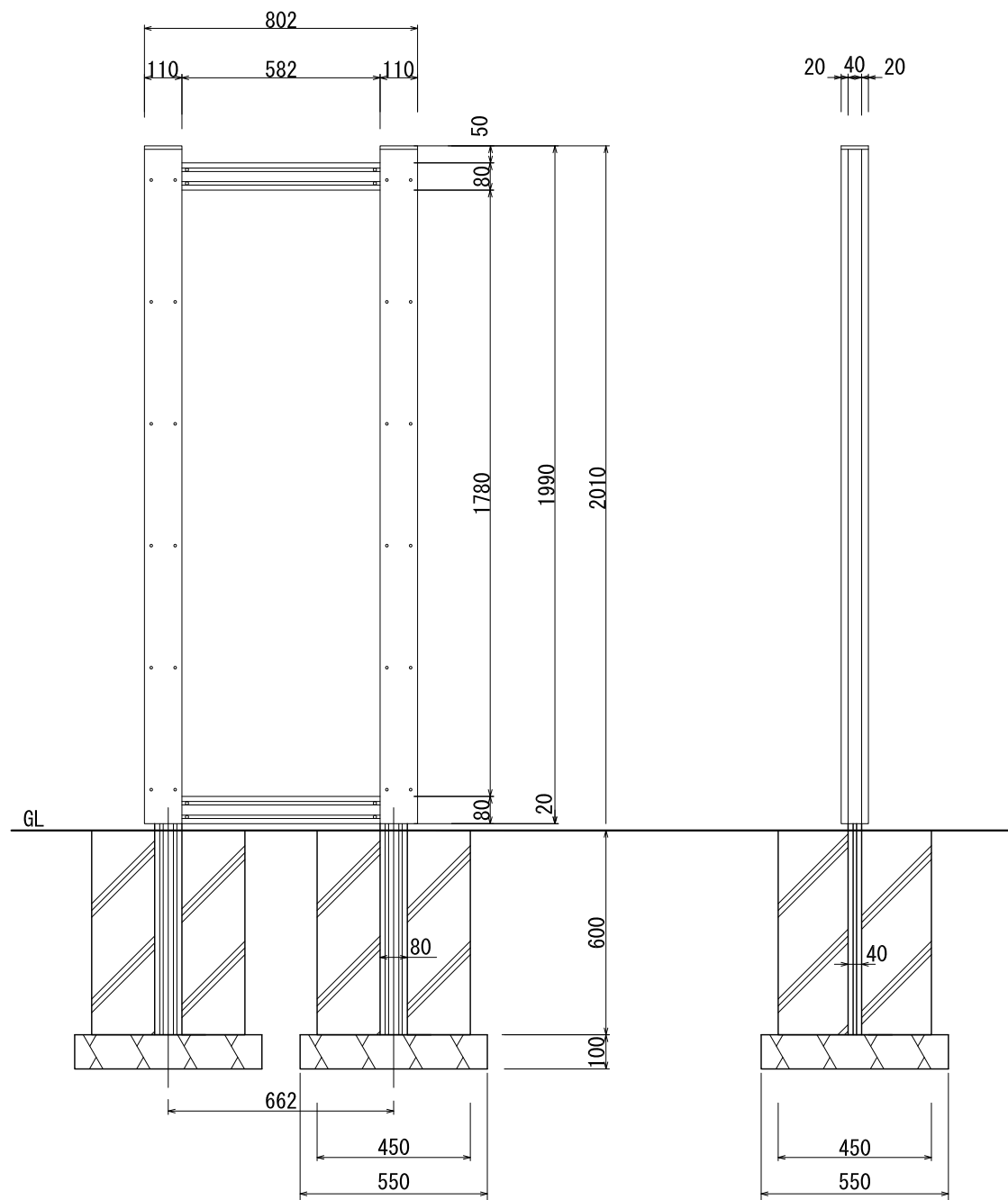
【正面図1:20】
