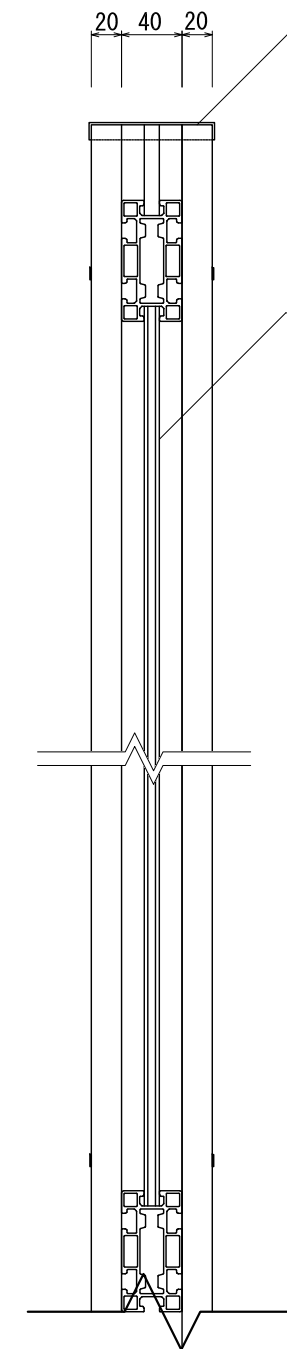
【側断面図1:5】
