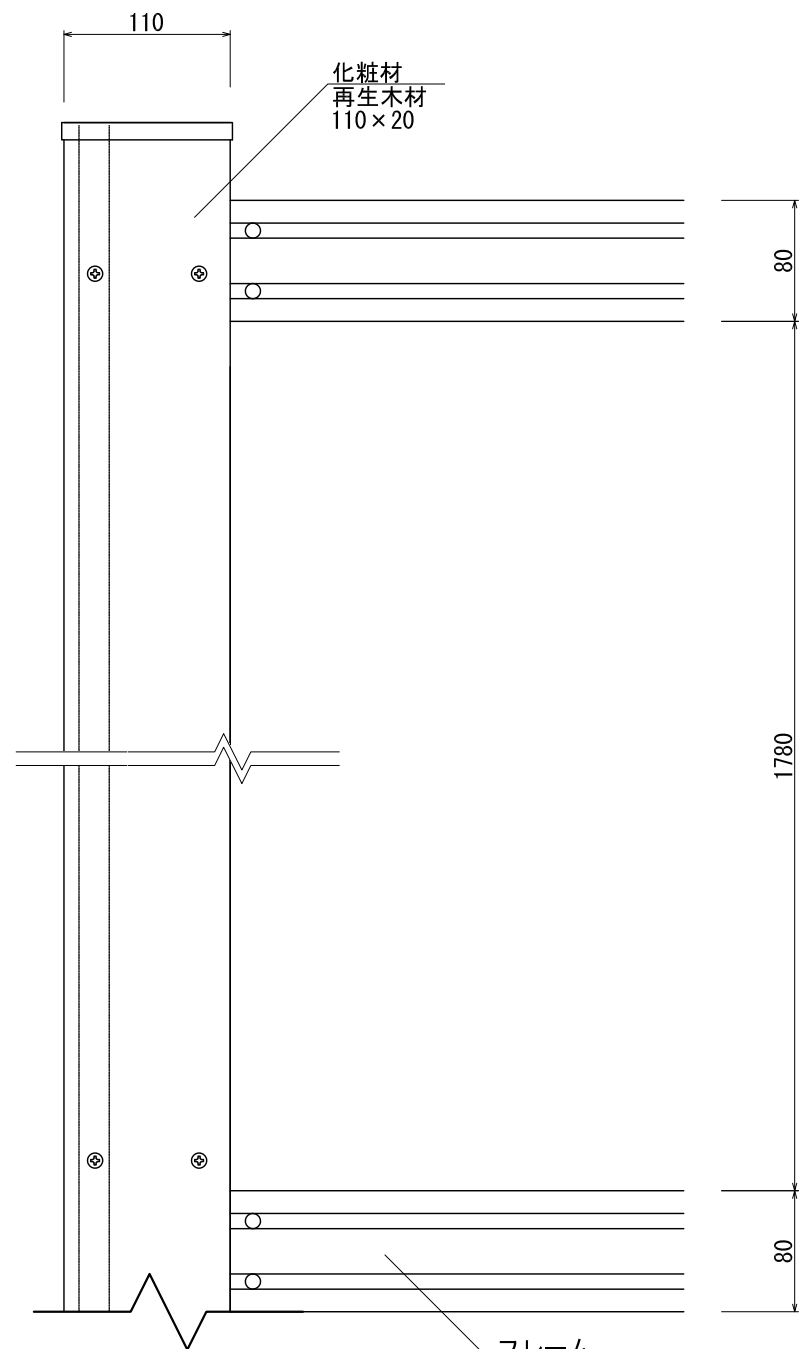
【正面図1:5】
