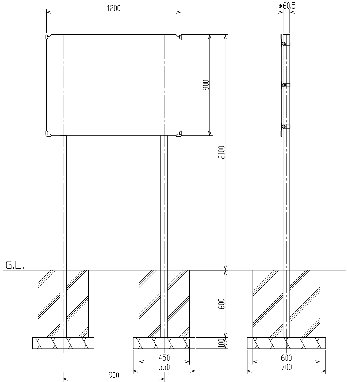
正面図 S = 1/20
