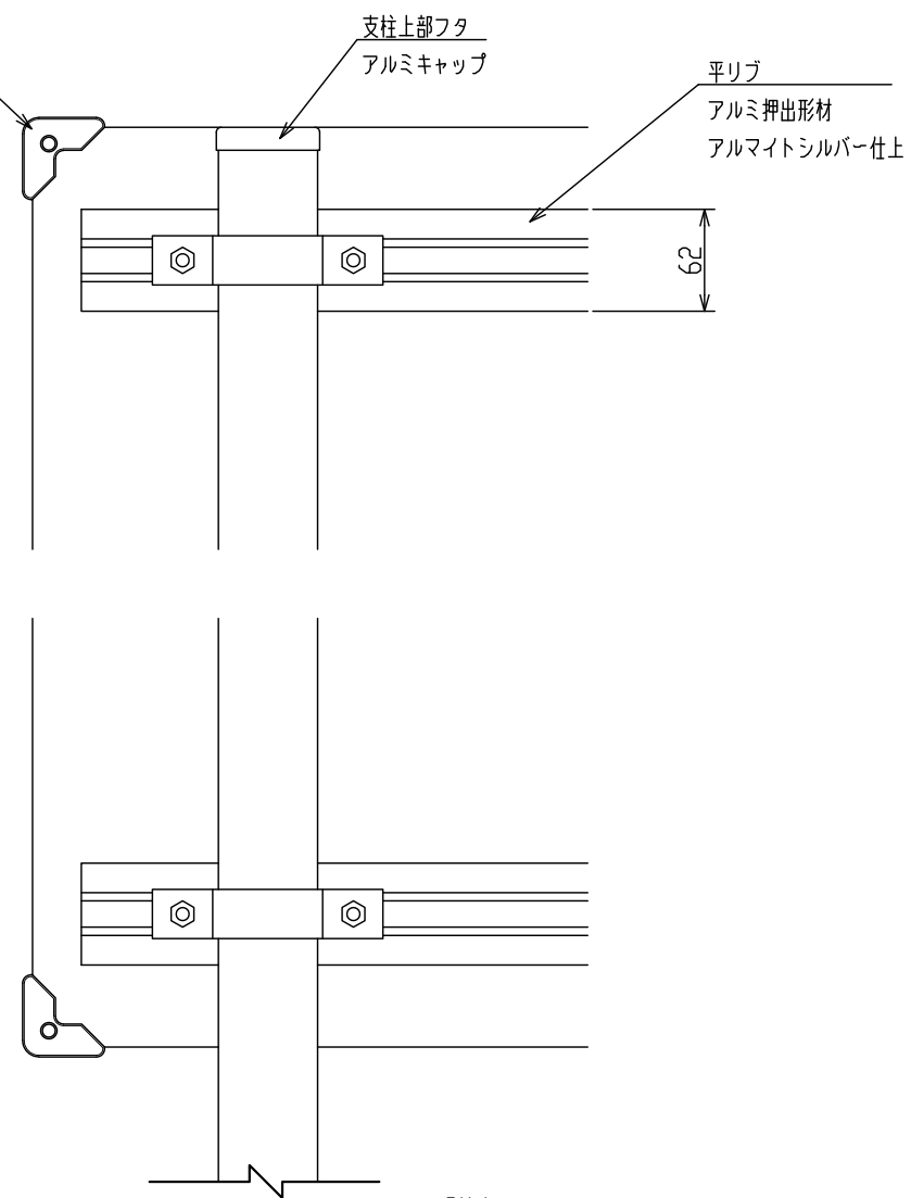
詳細図 S = 1/5
