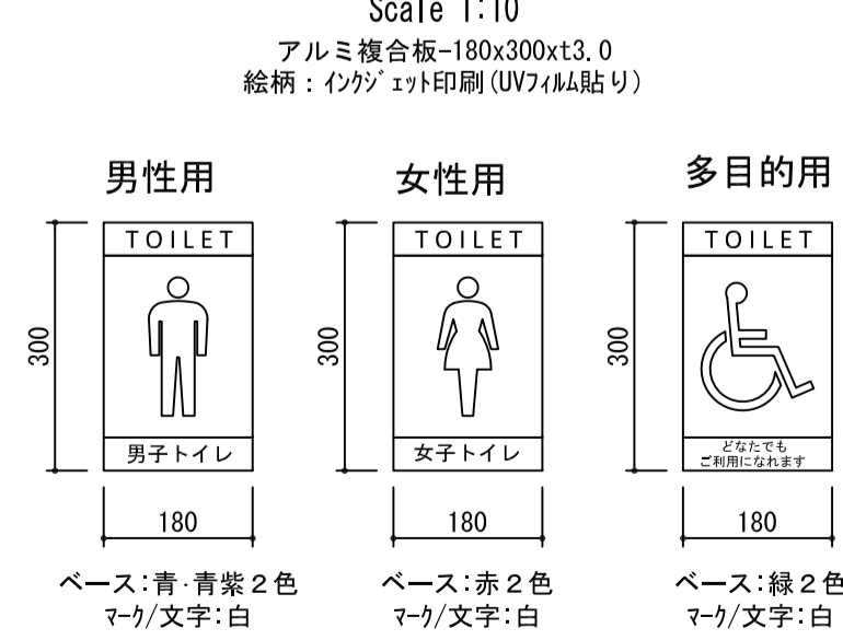
ピクトサイン詳細図 Scale 1:10
