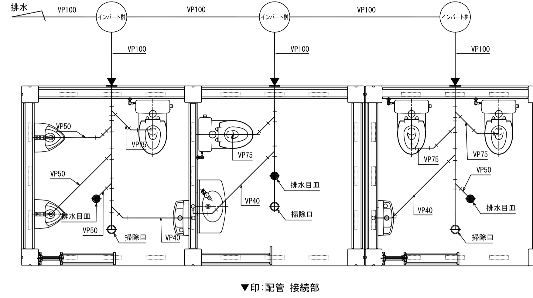
「排水」系統参考図
