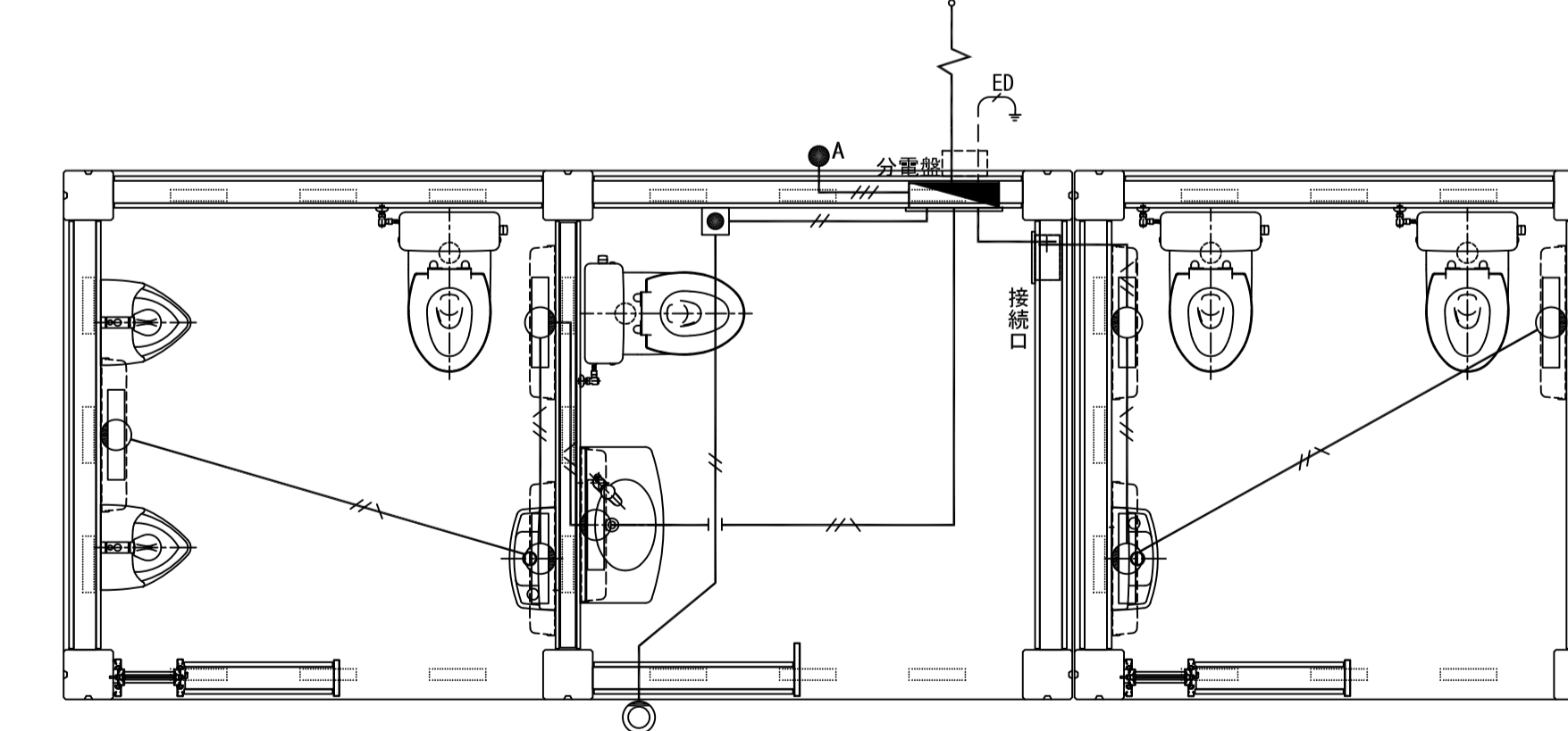
「電気」系統参考図
