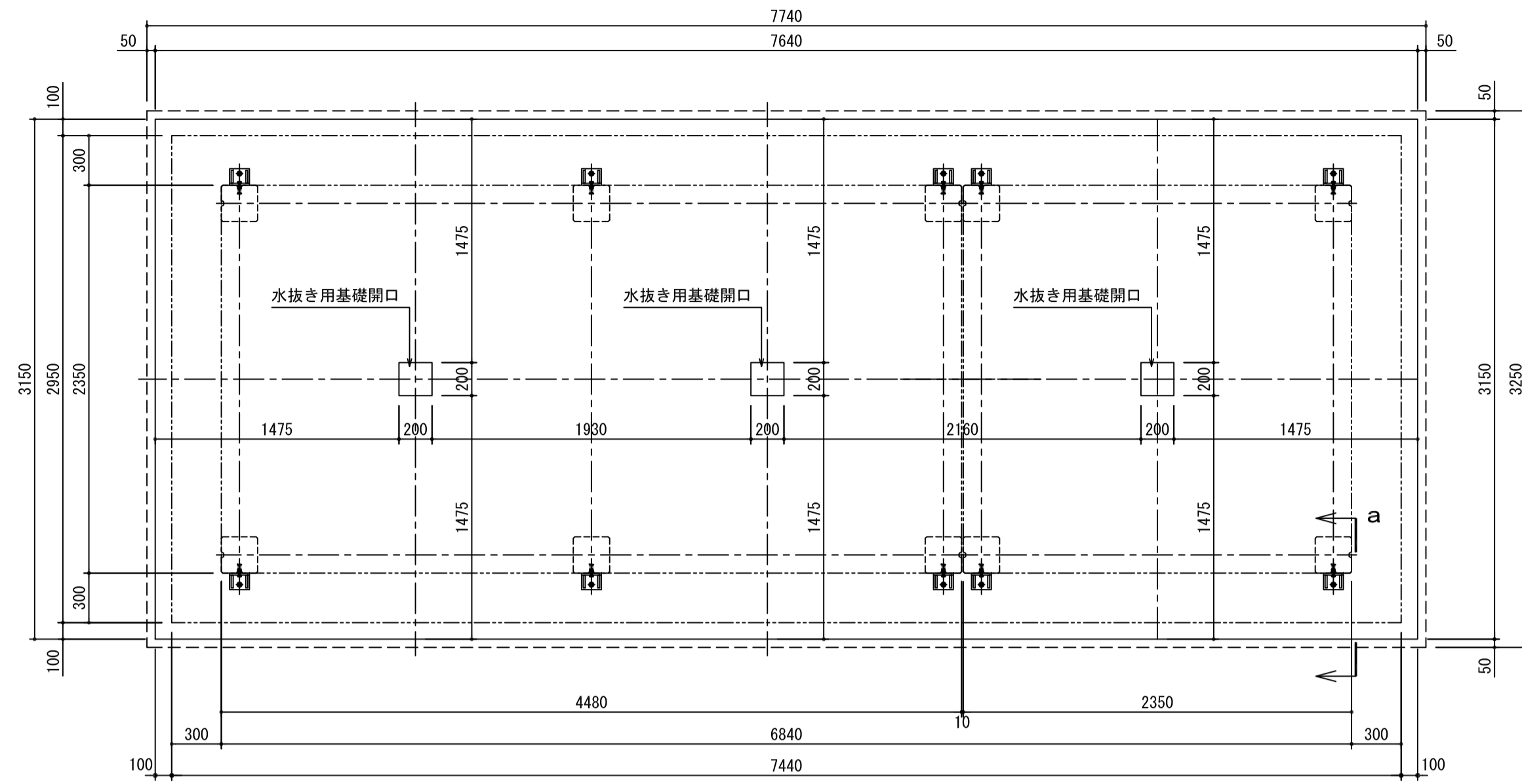
ベースコンクリート伏図
