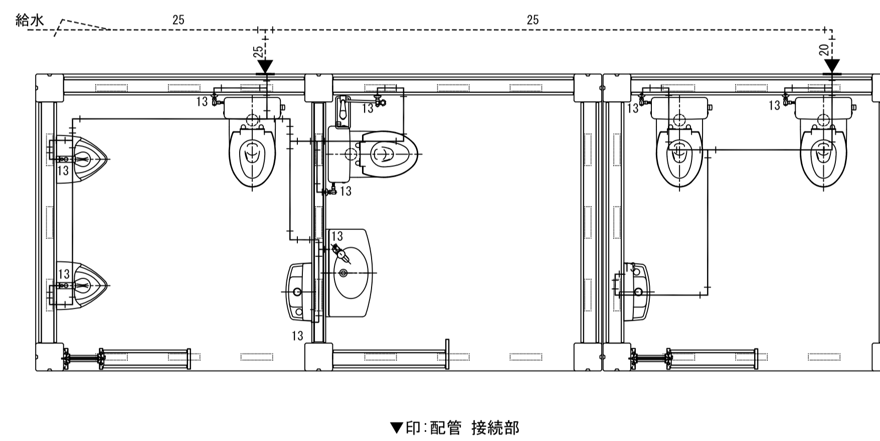
「給水」系統参考図
