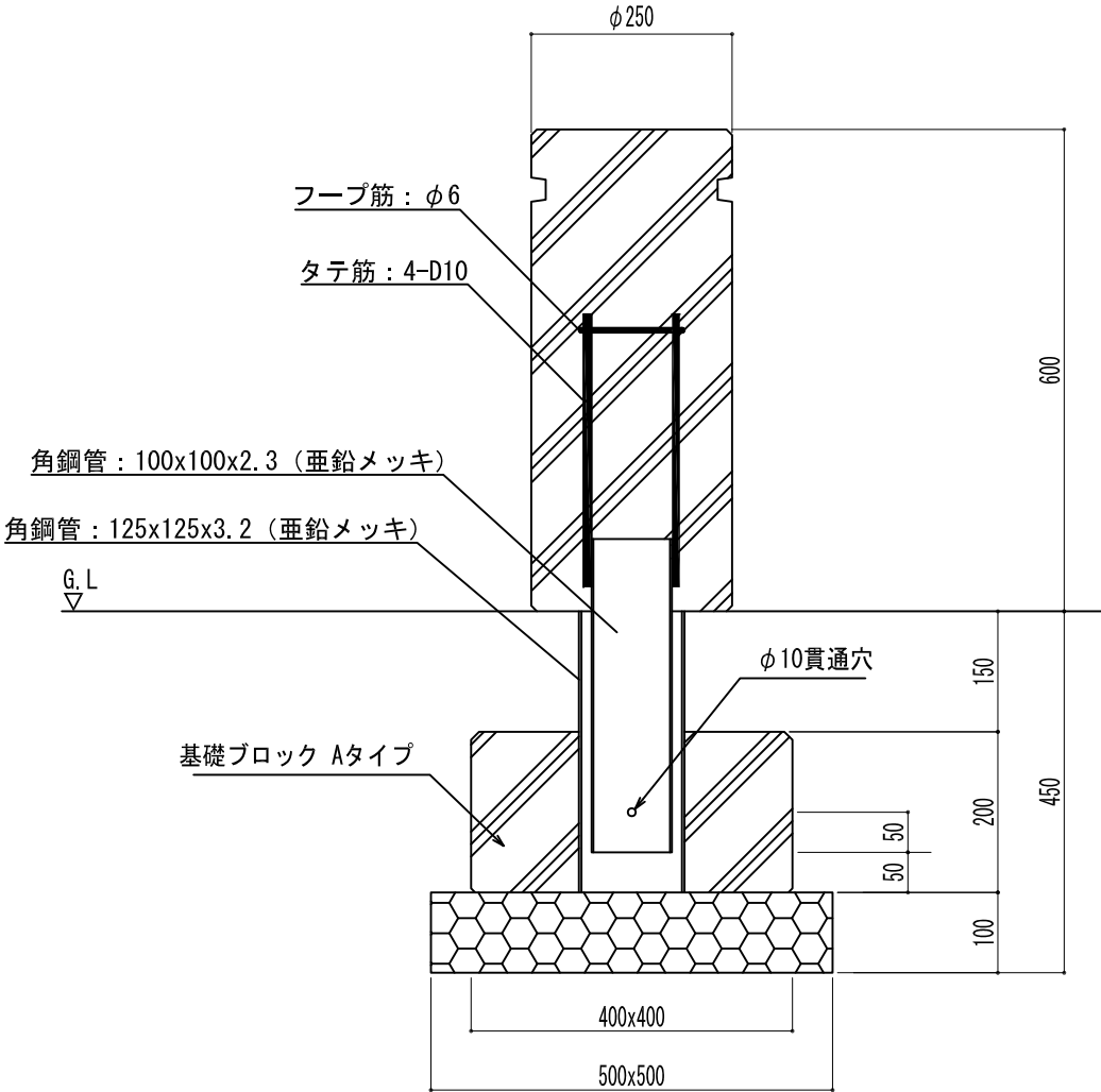
断面図
