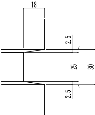
目地部詳細図 Scale 1:2
