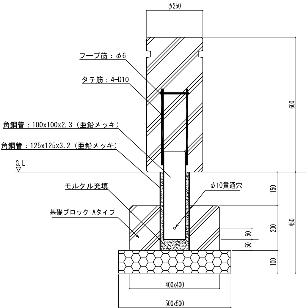
断面図
