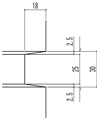
目地部詳細図
