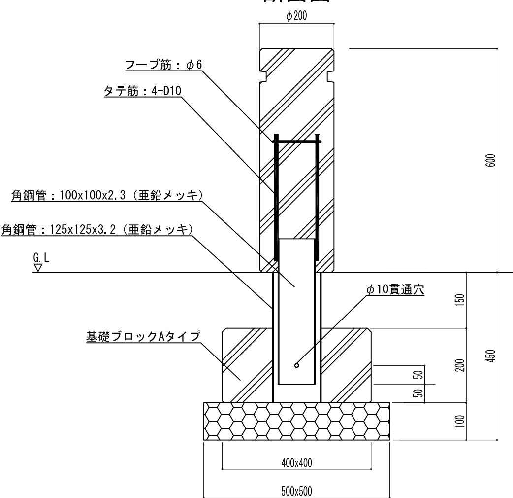
断面図
