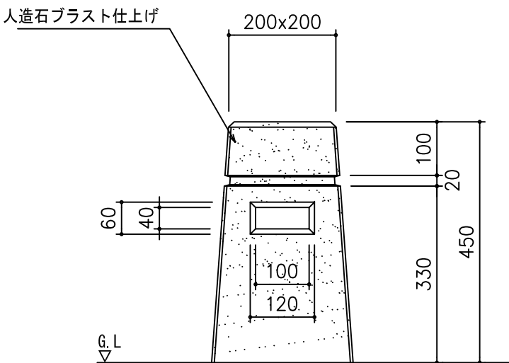
正面図
