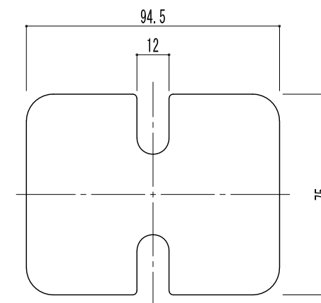
アンカー取付部分詳細図 S=1/2
