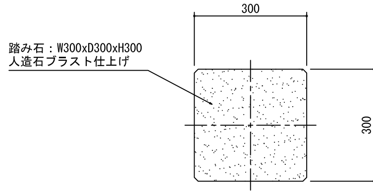
平面図
