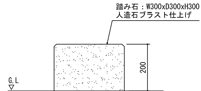
側面図
